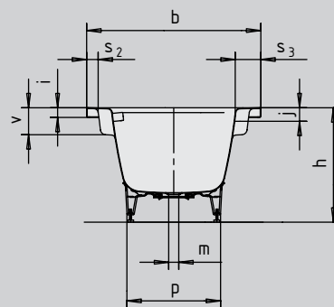
Расположение поручня
